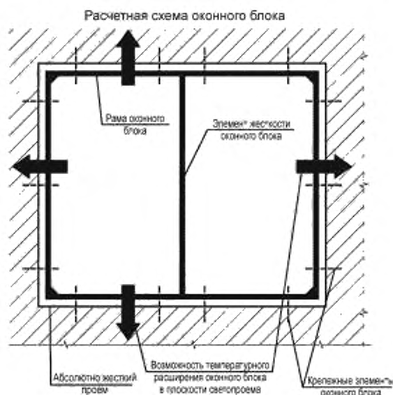
Рисунок 1 — Условия работы оконного блока
