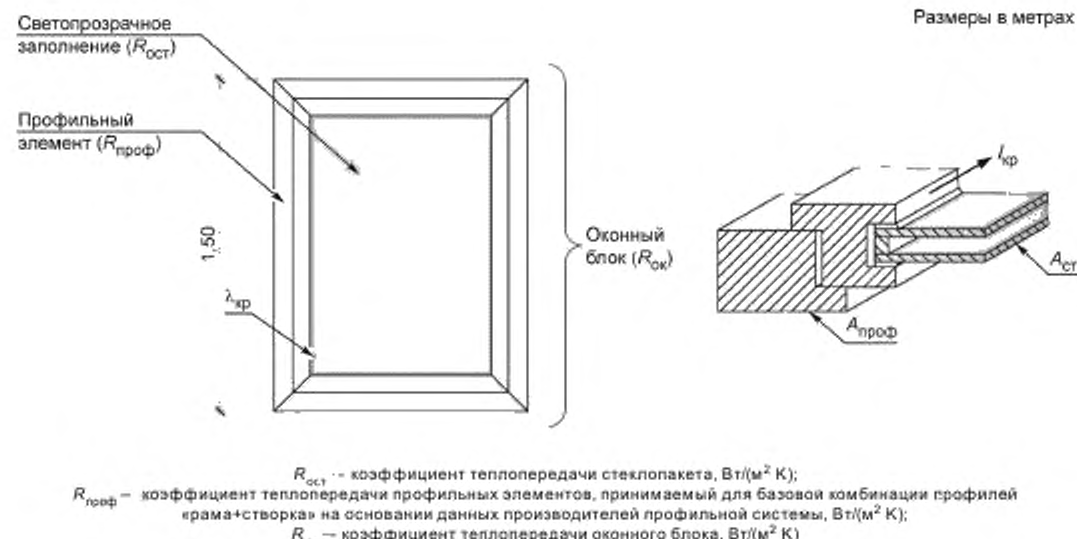
Рисунок А.1 — Расчетная схема для определения приведенного сопротивления теплопередаче оконных (балконных) блоков
