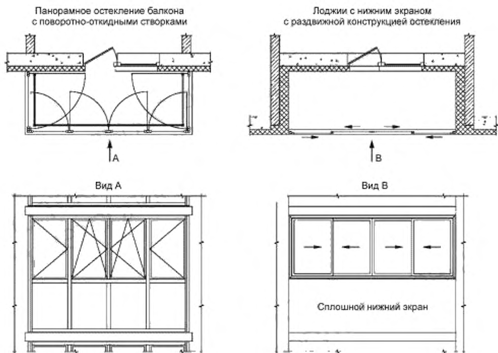
Рисунок Д.2 — Примеры конструкций наружного остекления
